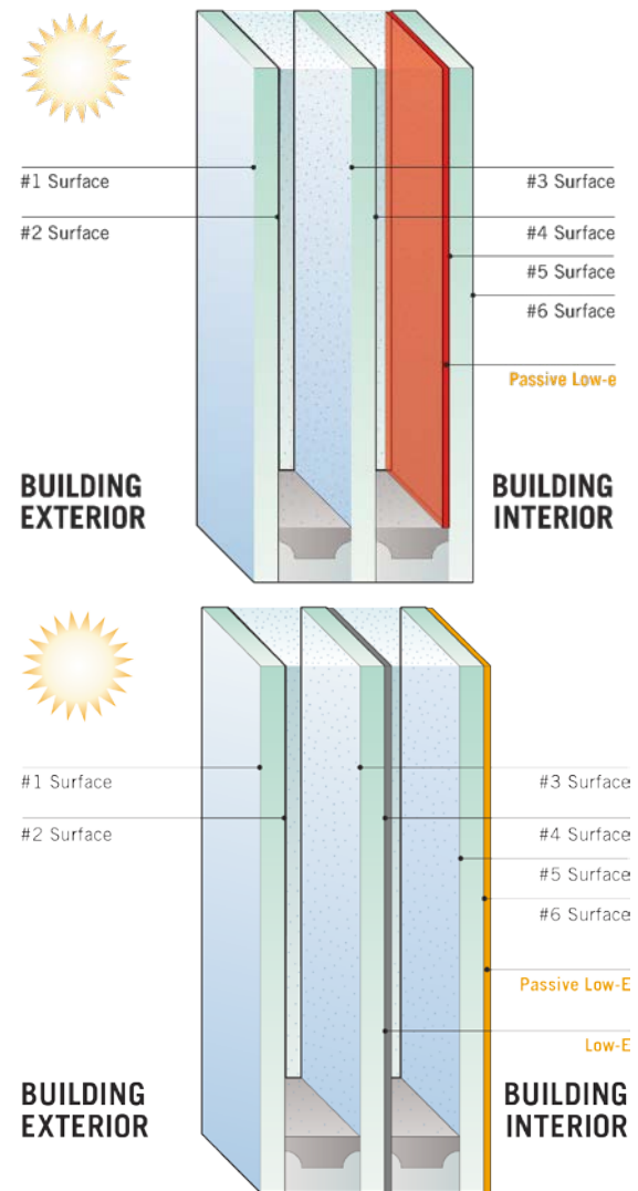
Triple-Pane IGU
